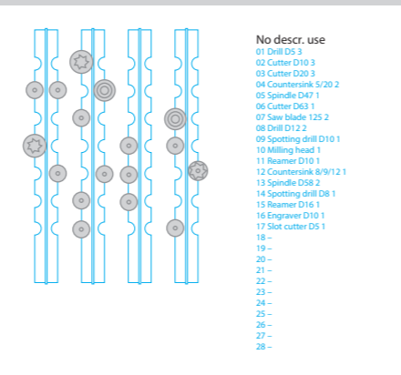
툴 교환리스트 »cetus« 사용 시
